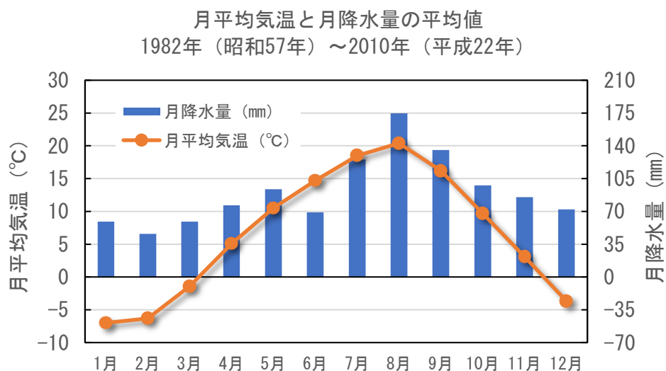
図1.3.5-3 気温、降水量の平均値 (1982（昭和57）年～2010（平成22）年）
