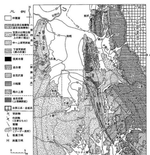
図1.3.5-2 馬追丘陵とその周辺の地質 破線内は千歳地区表層地質報告書の報告範囲。
